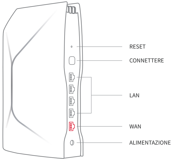
Configurazione porte
